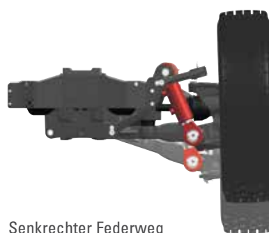
Senkrechter Federweg
